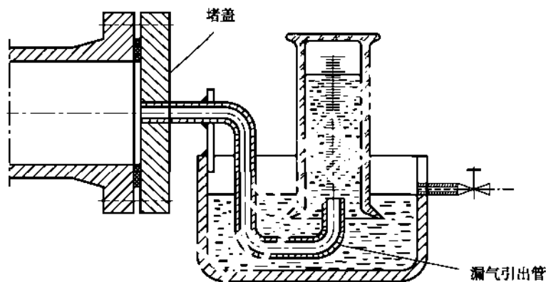
图 dc-4 排液集气检漏装置
