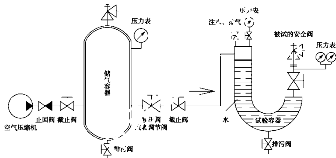
图 dc-2 推荐的液体介质安全阀校验装置
