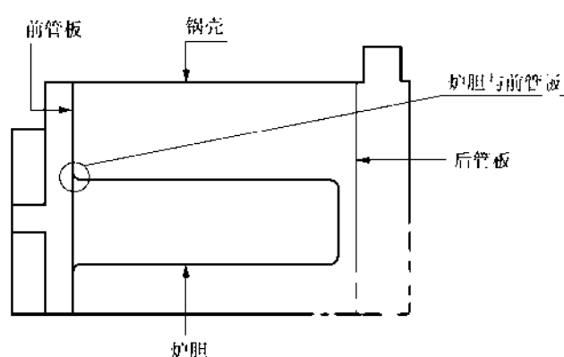
(c) 回燃式
