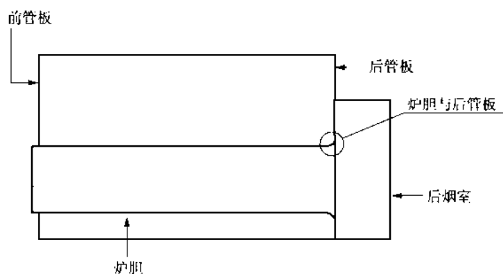
(b) 干背式
